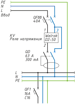
Схема 1. Вариант электрической схемы
