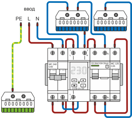
Схема 2. Вариант монтажной схемы
