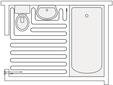
Пример укладки кабеля в помещении ванной комнаты
