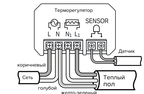
Подключение к 2-х проводной линии
