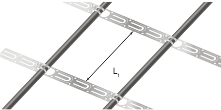
Шаг укладки кабеля на монтажной ленте
